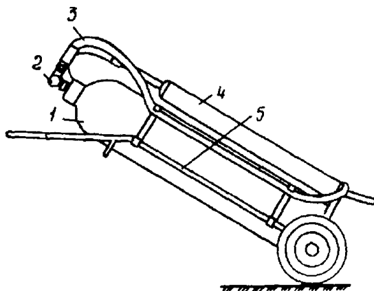
Передвижной углекислотный огнетушитель ОУ-25 и ОУ-80 состоит: 1 - баллон; 2 - запорный вентиль; 3 - шланг; 4 - раструб; 5 - тележка
