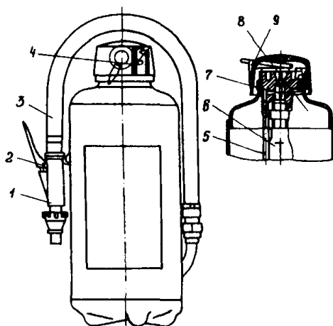
Переносной порошковый огнетушитель ОП-5 состоит: 1 - пистолет; 2 - рычаг; 3 - рукав; 4 - пломба; 5 - сифонная труба; 6 - баллончик; 7 - игла; 8 - корпус; 9 - чека
