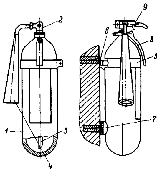
Переносной углекислотный огнетушитель ОУ-5 (ОУ-8) состоит: 1 - баллон; 2 - поворотный раструб; 3 - запорная головка; 4 - сифонная трубка; 5 - хомут; 6 - крюк; 7 - упор; 8 - ручка; 9 - чека
