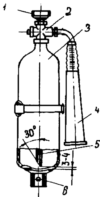
Переносной углекислотный огнетушитель ОУ-2 состоит: 1 - маховичок; 2 - вентиль; 3 - баллон; 4 - раструб; 5 - сифонная трубка; 6 - кронштейн
